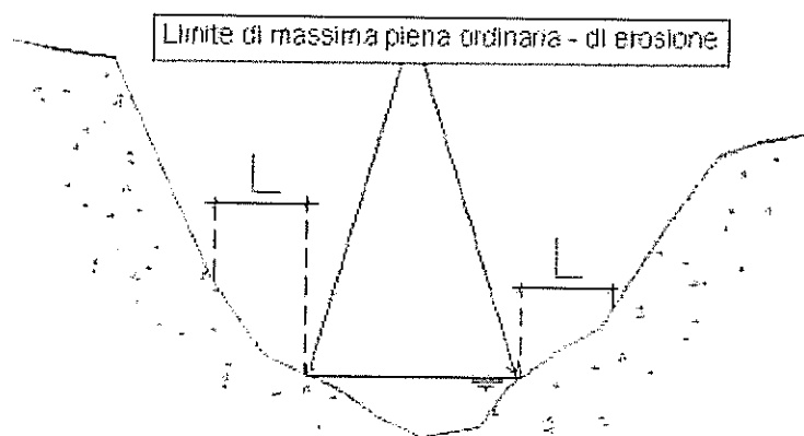
CORSO D'ACQUA PRIVO DI ARGINATURA CON SEZIONE BAGNATA MOLTO PICCOLA RISPETTO ALLA SEZIONE DEL VALLETTO
