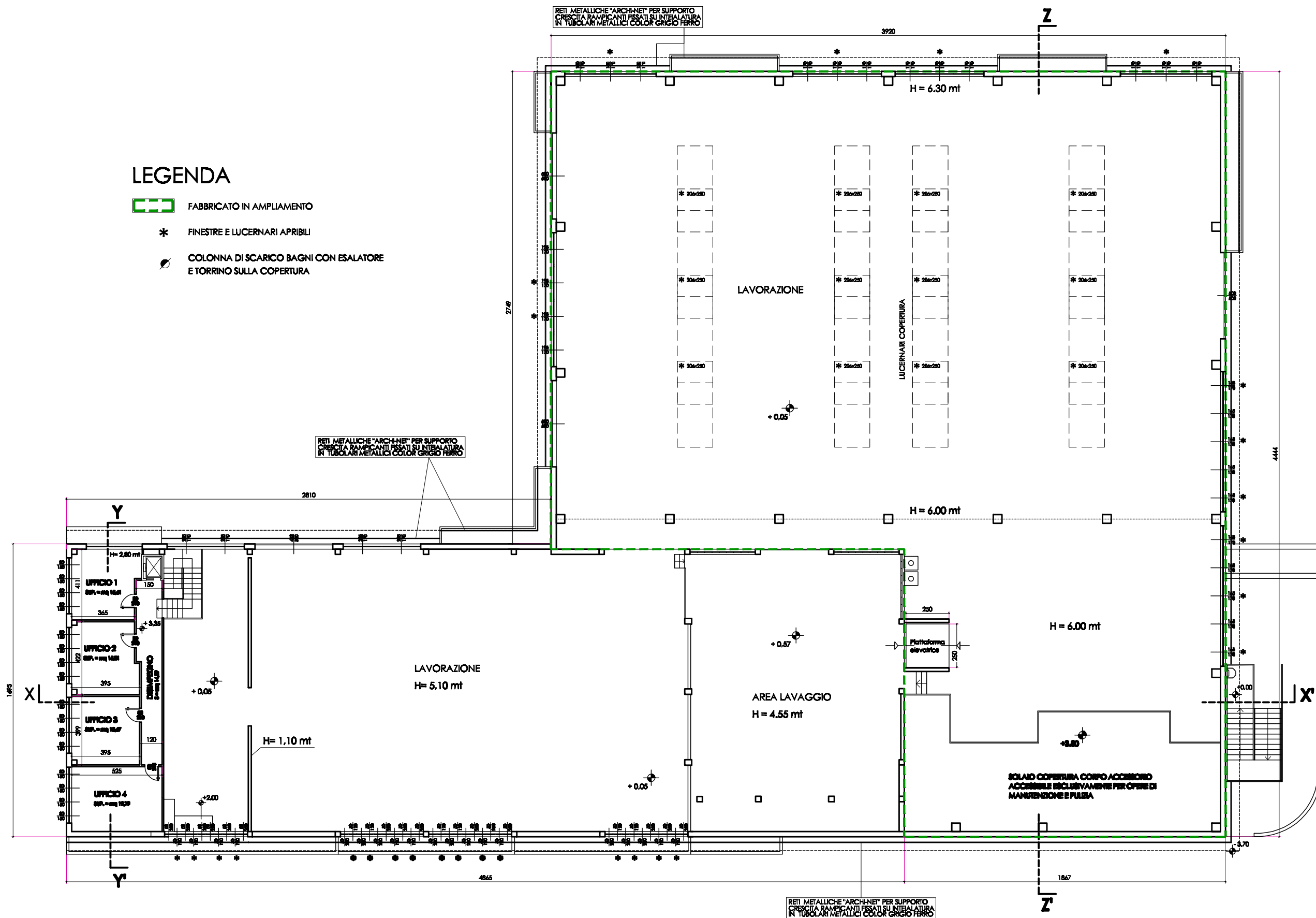
TAV. 08 - PIANTA PIANO TERRA - PROGETTO (quota + 4.00)
